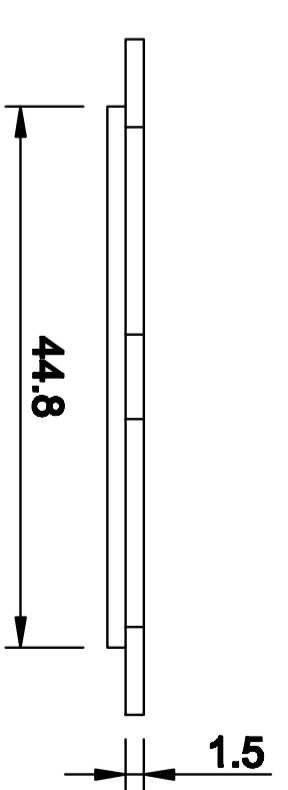
FAN GUARD
